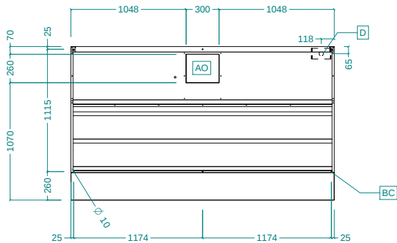
Вид сверху
