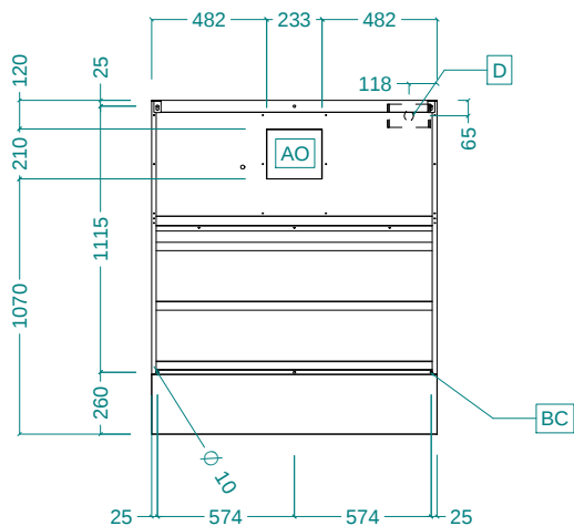
Вид сверху
