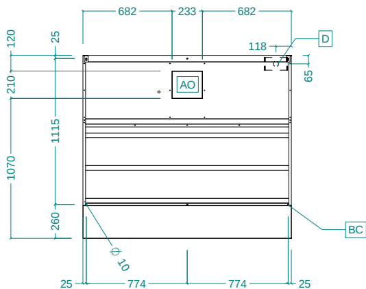
Вид сверху
