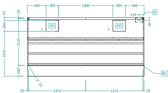
Вид сверху
