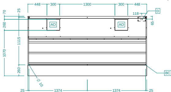
Вид сверху
