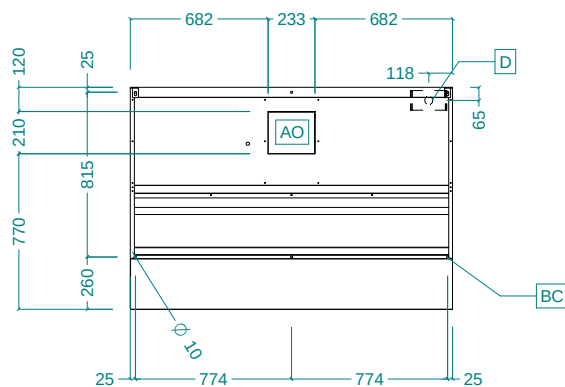
Вид сверху
