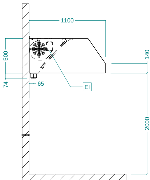
Вид сбоку
