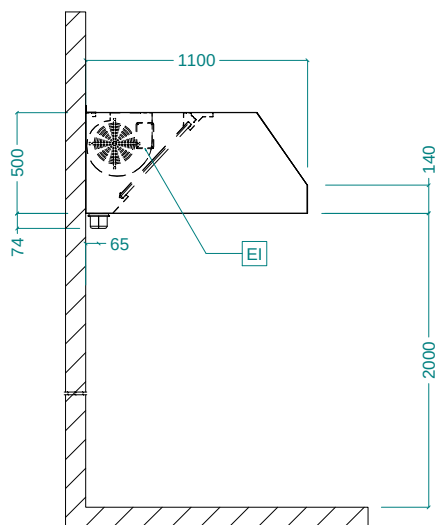
Вид сбоку
