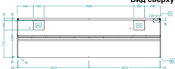
Вид сверху
