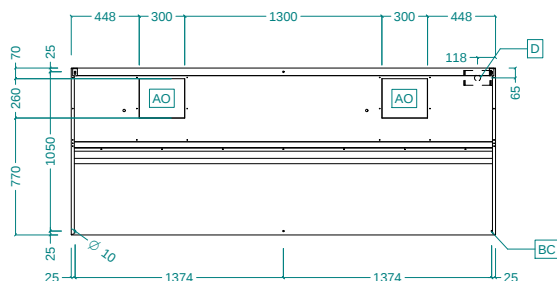
Вид сверху
