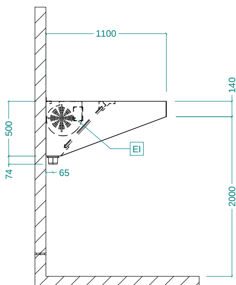
Вид сбоку
