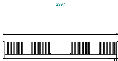
Вид спереди
