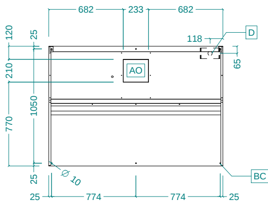
Вид сверху
