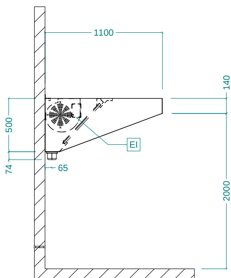
Вид сбоку
