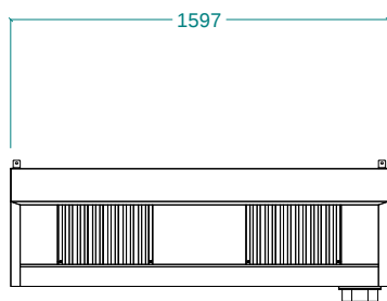
Вид спереди
