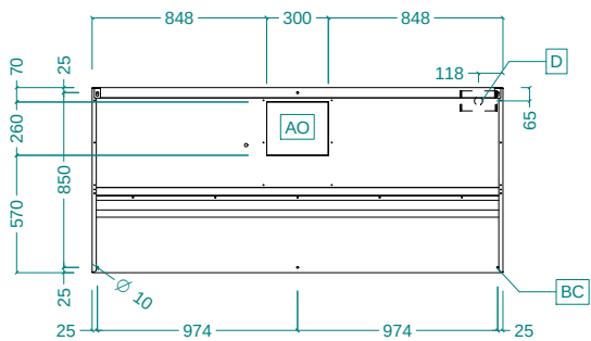
Вид сверху
