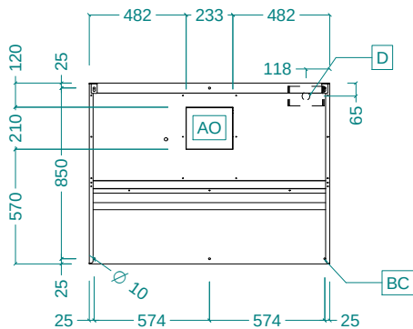
Вид сверху
