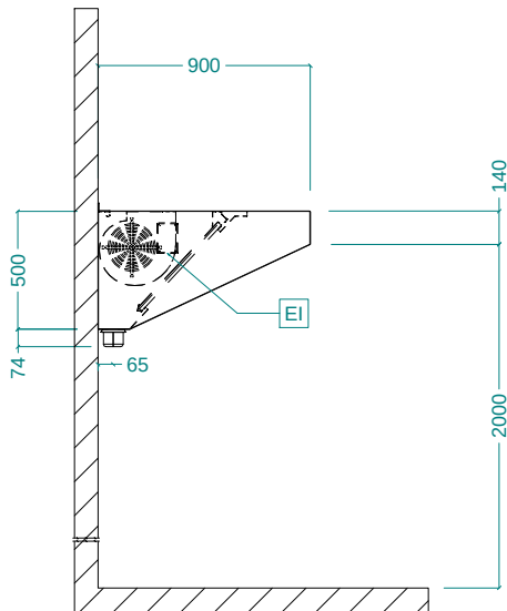
Вид сбоку
