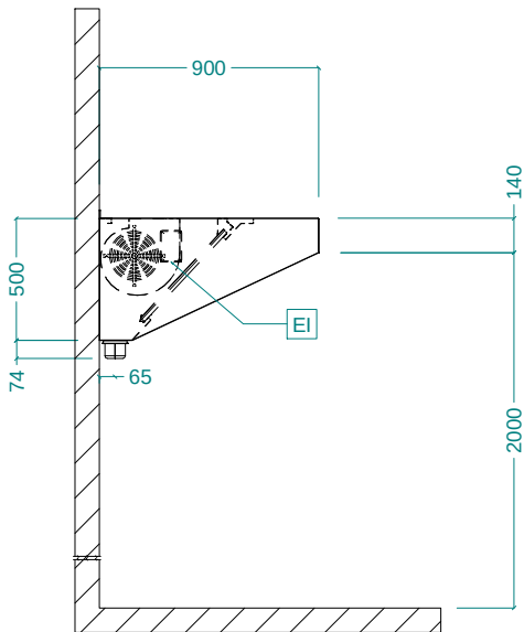
Вид сбоку
