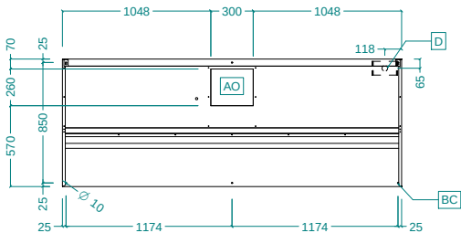
Вид сверху
