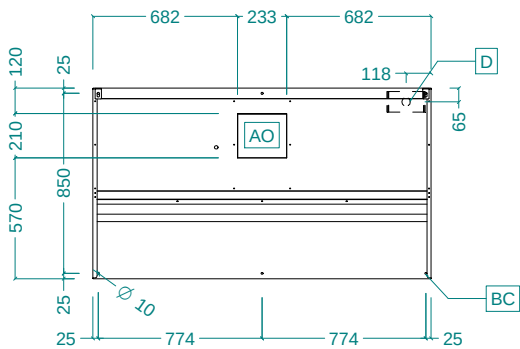
Вид сверху
