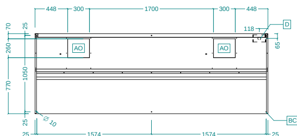
Вид сверху
