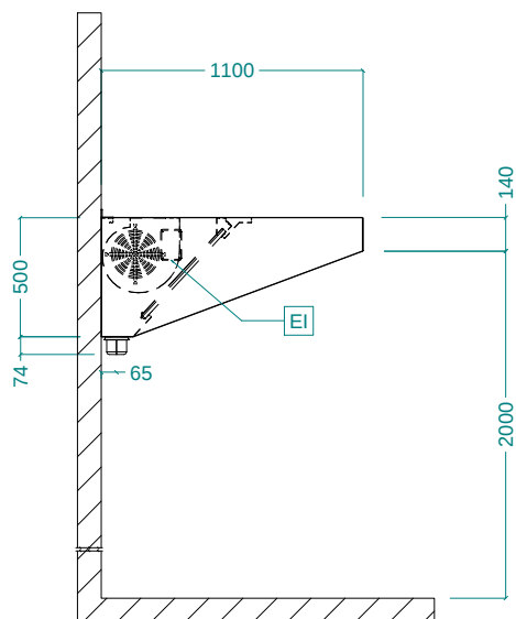
Вид сбоку
