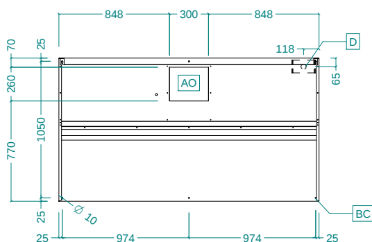
Вид сверху
