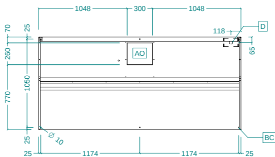
Вид сверху
