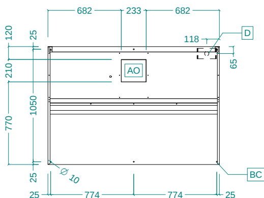
Вид сверху
