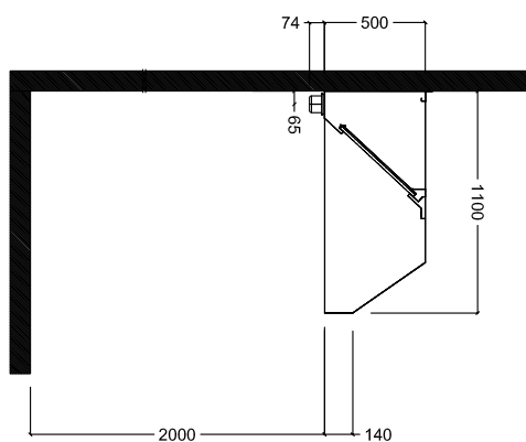
Вид сбоку
