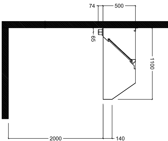
Вид сбоку
