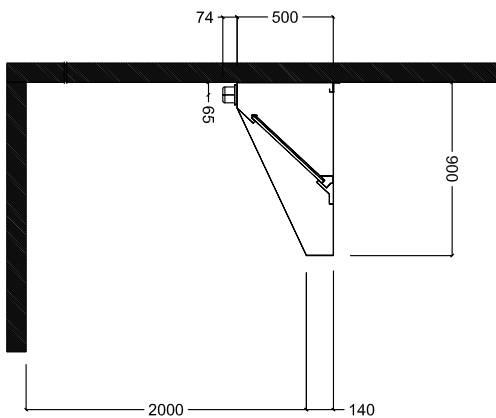
Вид сбоку
