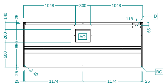
Вид сверху
