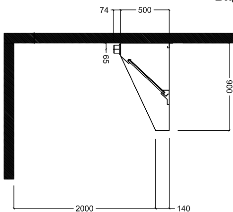
Вид сбоку
