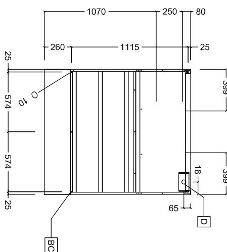
Вид сверху
