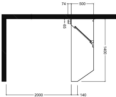
Вид сбоку
