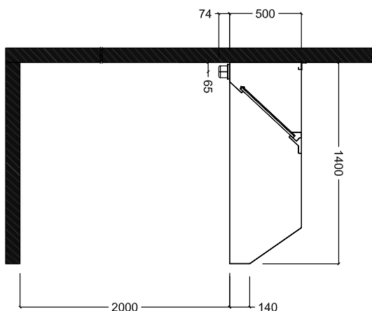
Вид сбоку
