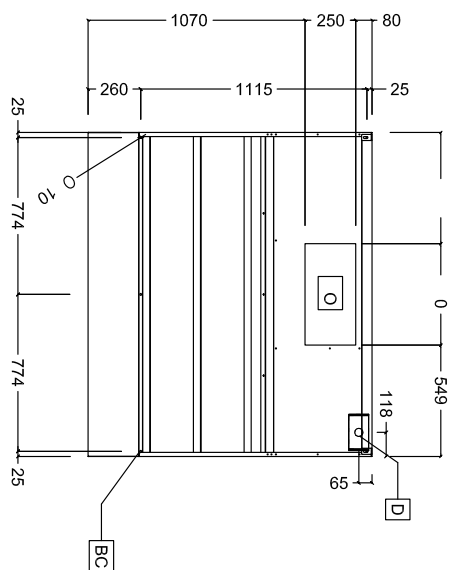
Вид сверху
