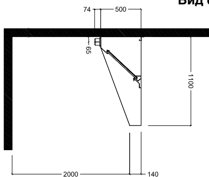
Вид сбоку
