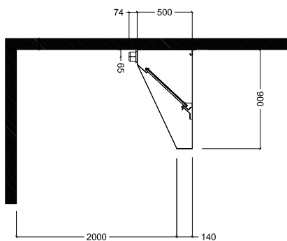
Вид сбоку
