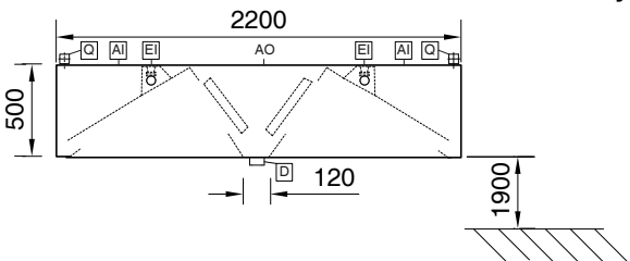
Вид сбоку
