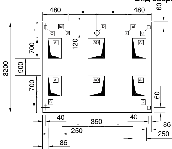
Вид сверху
