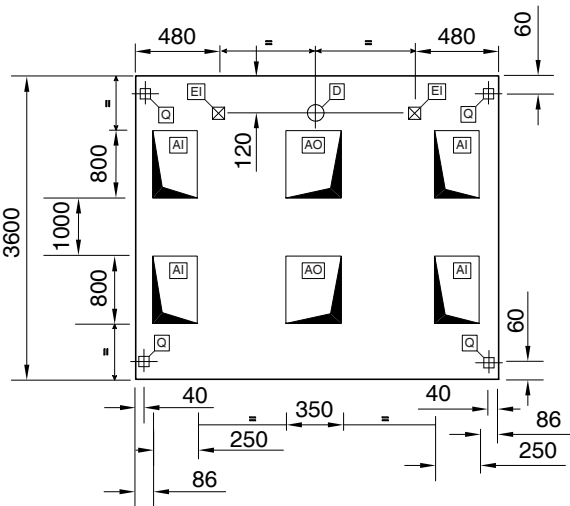
Вид сверху
