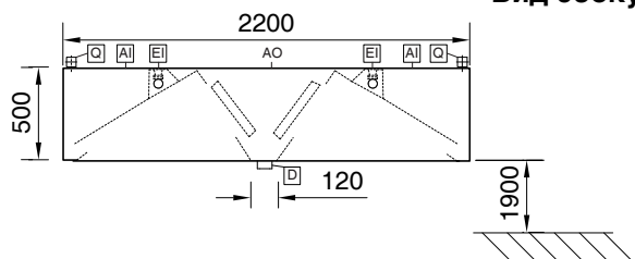
Вид сбоку
