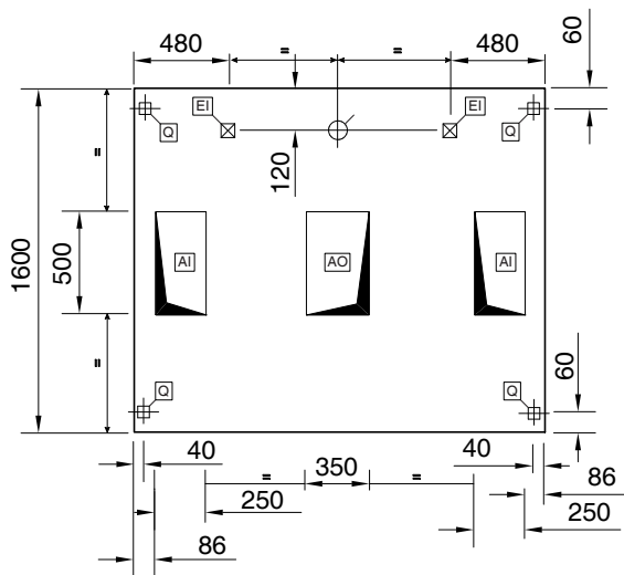
Вид сверху
