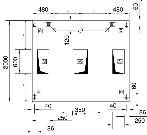
Вид сверху
