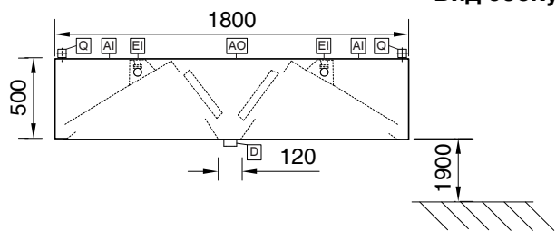
Вид сбоку
