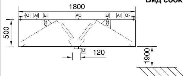
Вид сбоку
