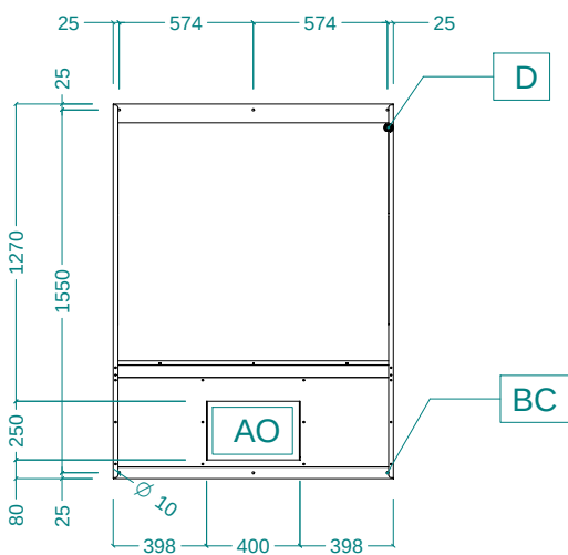
Вид сверху
