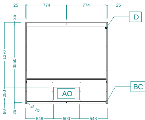
Вид сверху
