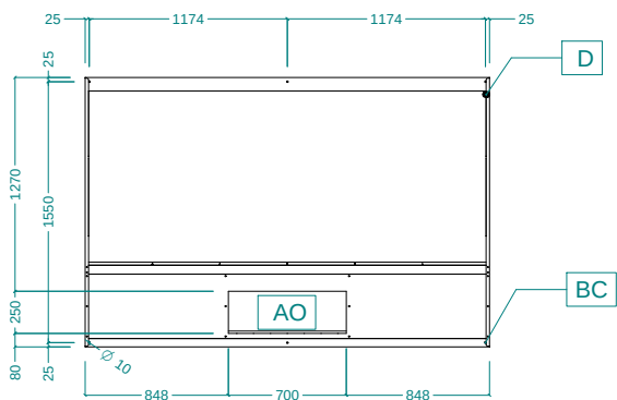
Вид сверху
