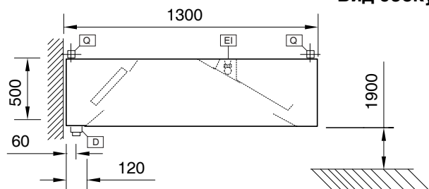
Вид сбоку
