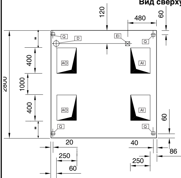
Вид сверху
