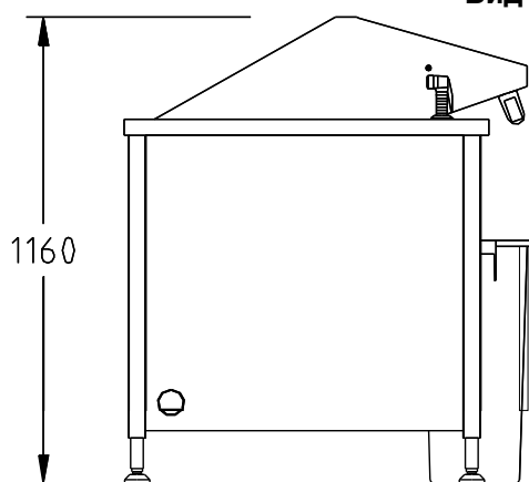
Вид сбоку
