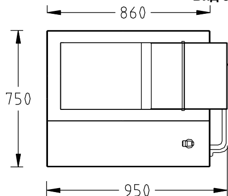
Вид сверху
