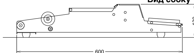
Вид сбоку
