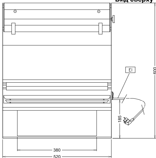
Вид сверху
