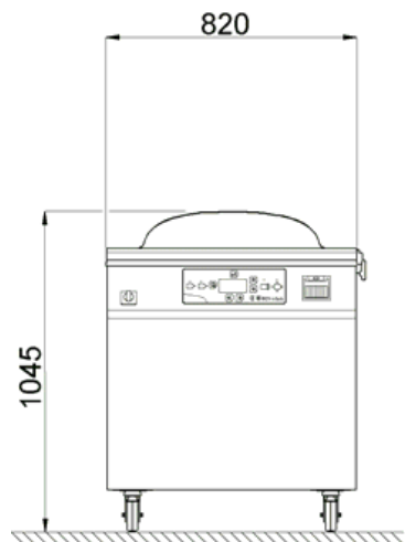
Вид спереди
