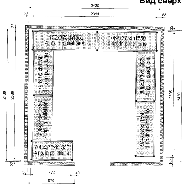
Вид сверху
