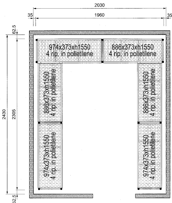
Вид сверху
