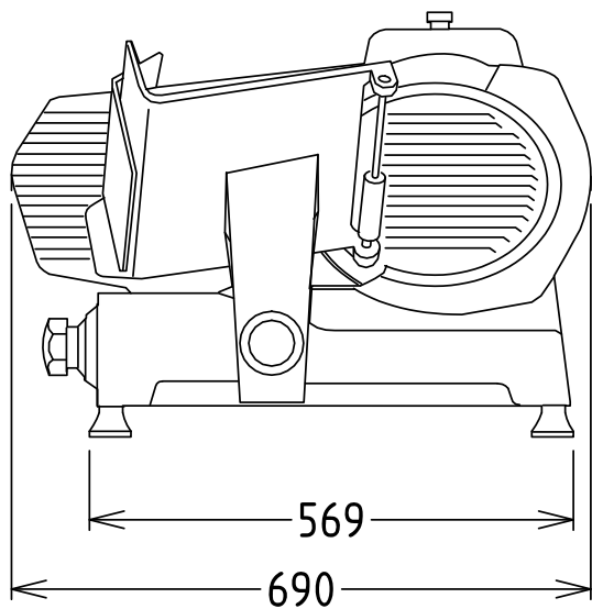
Вид спереди
