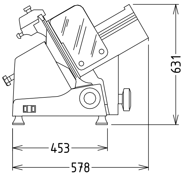
Вид сбоку
