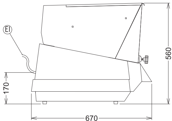
Вид сбоку
