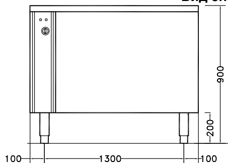
Вид спереди
