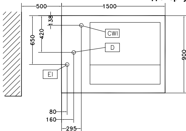
Вид сверху
