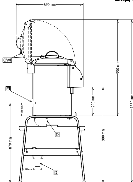
Вид сбоку
