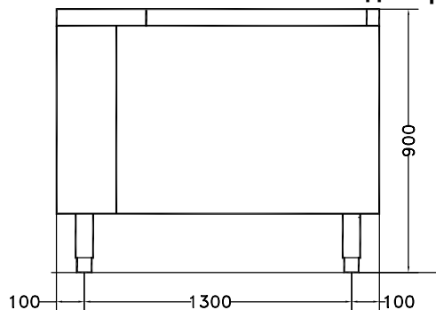
Вид спереди
