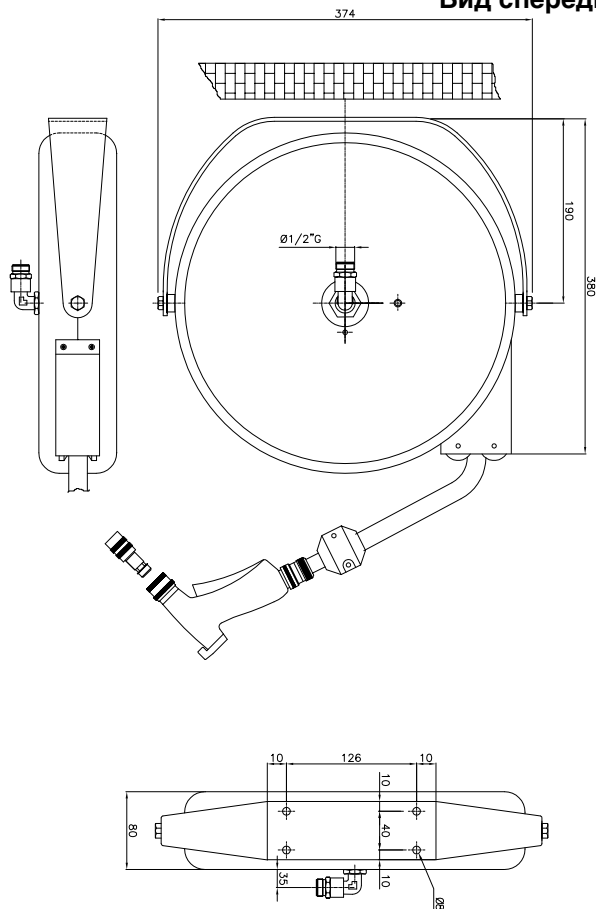
Вид спереди
