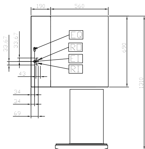
Вид сверху
