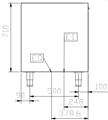
Вид сбоку
