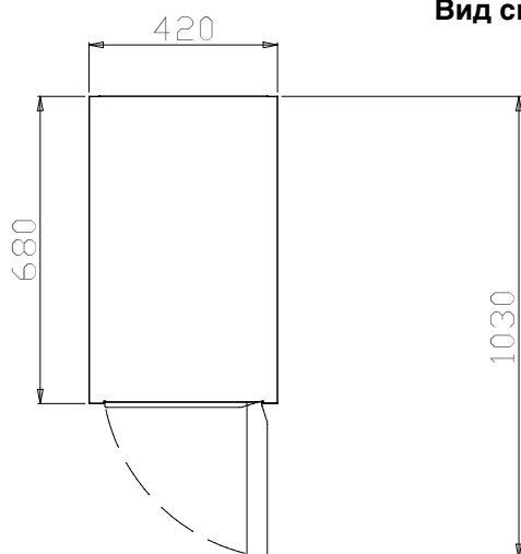
Вид сверху
