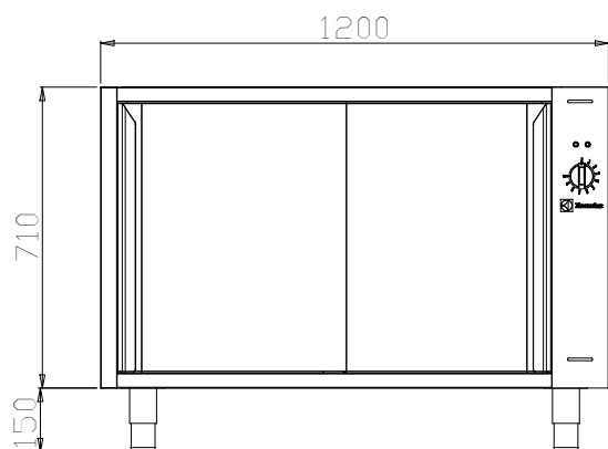
Вид спереди
