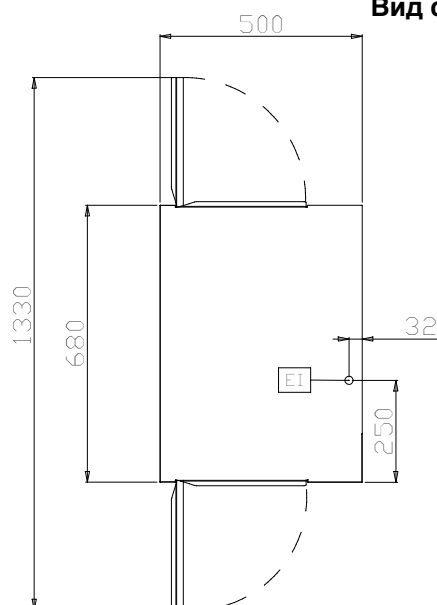
Вид сверху
