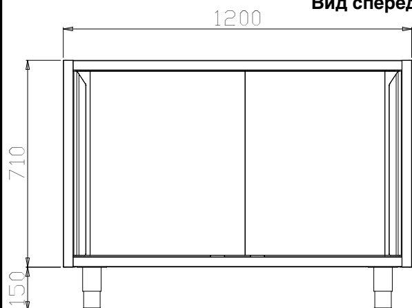
Вид спереди
