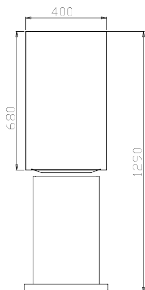
Вид сверху
