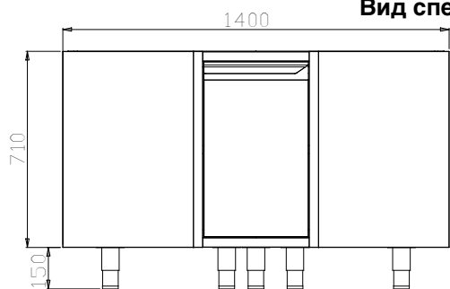
Вид сбоку
