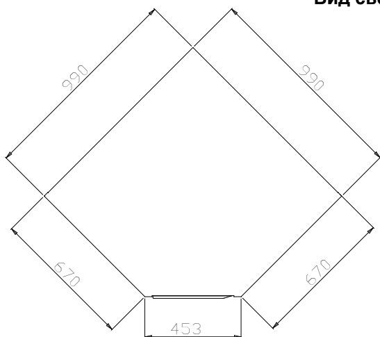
Вид сверху
