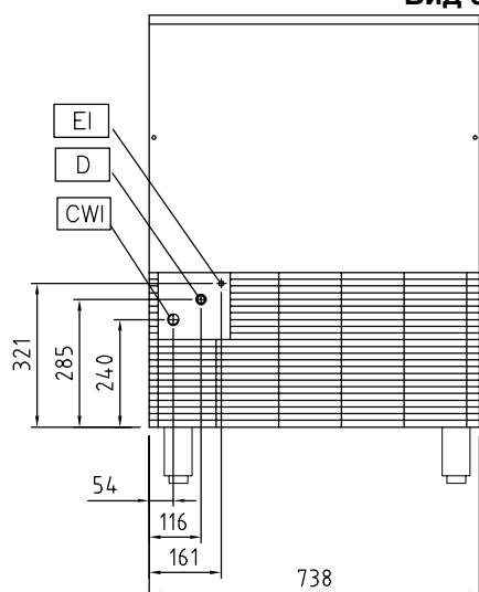
Вид спереди
