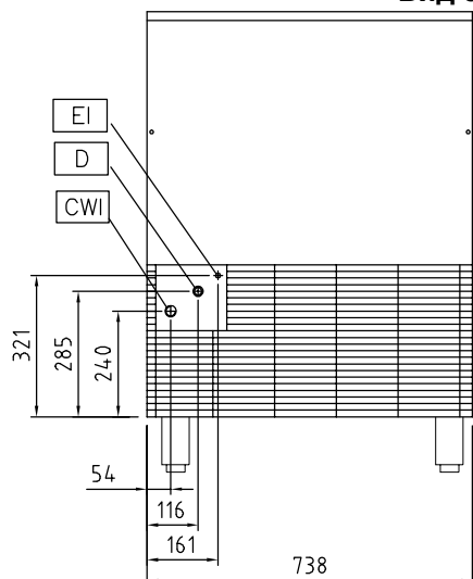
Вид спереди
