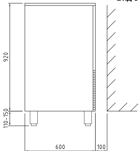
Вид сбоку
