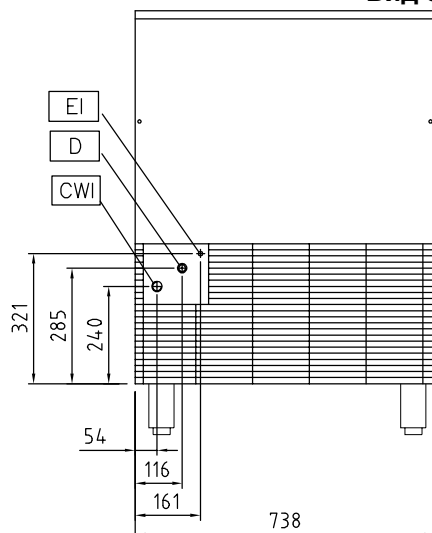
Вид спереди
