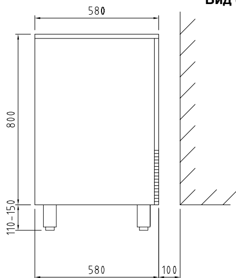
Вид сбоку
