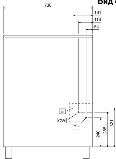
Вид спереди
