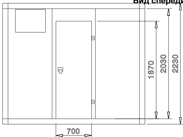
Вид спереди
