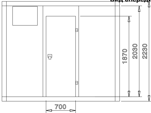
Вид спереди
