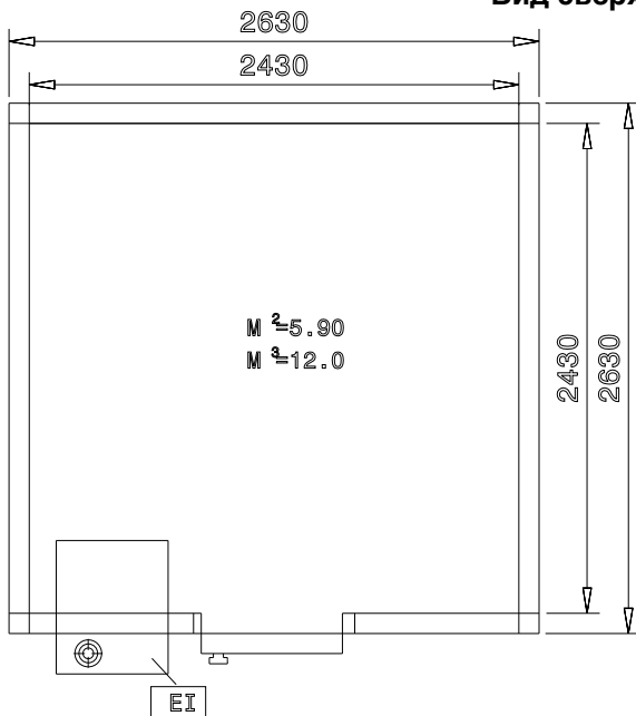
Вид сверху
