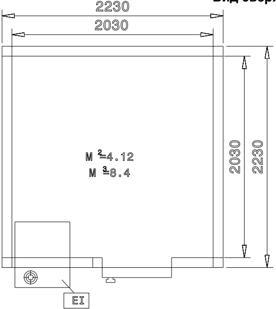
Вид сверху
