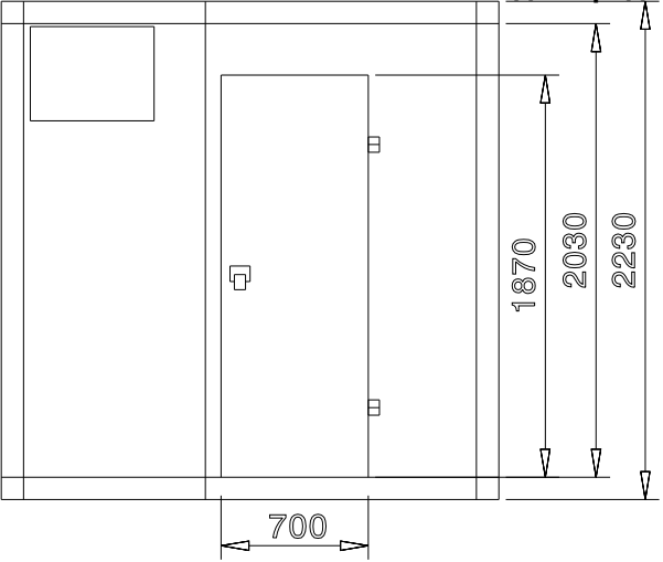
Вид спереди
