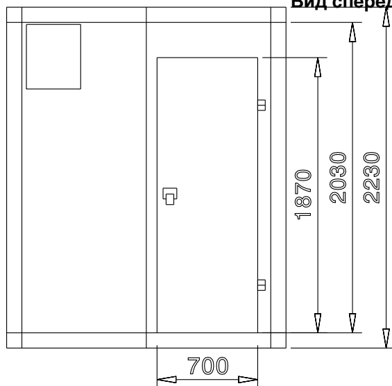
Вид спереди
