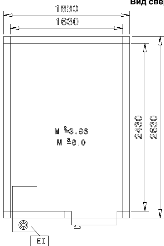
Вид сверху
