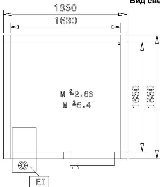
Вид сверху
