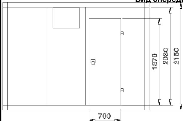
Вид спереди
