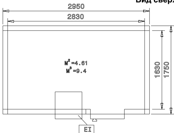
Вид сверху
