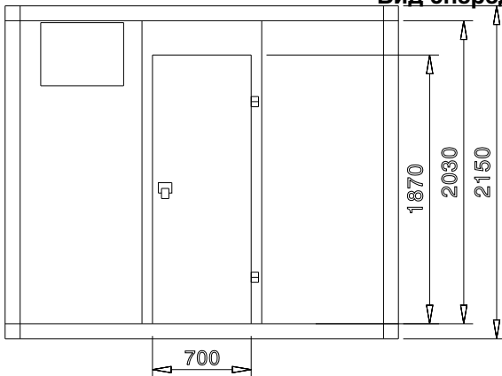
Вид сбоку
