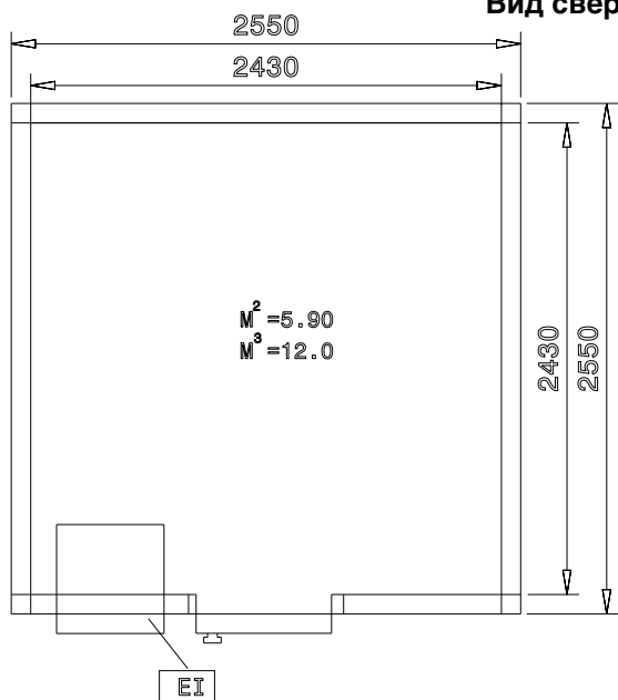
Вид сверху
